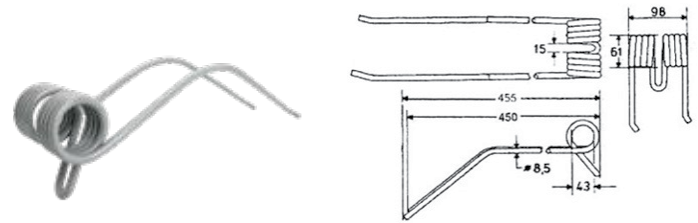
CLAAS LINER VOLTO RAKE TINE CLAAS 9568151 45.000.700
